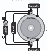
Mabuchi motor
